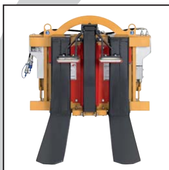
Forche in posizione chiusa Forks in closed position
